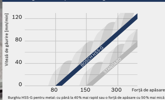
Viteză de găurire comparativ cu burghiile HSS-R standard
